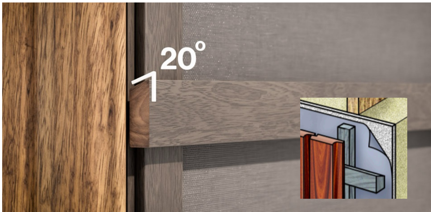
Afbeelding 4: Dubbel regelwerk bij verticale montage met correcte afschuining richting de spouw
