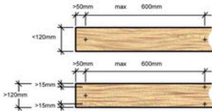
Maatvoering bevestigingspunten.
